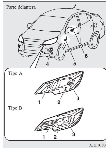
Tipo A: tipo de faros delanteros de halógeno Tipo B: tipo de faros de LED
